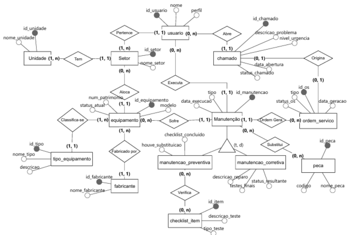
Figura 1: Modelo Conceitual (Diagrama Entidade-Relacionamento)
